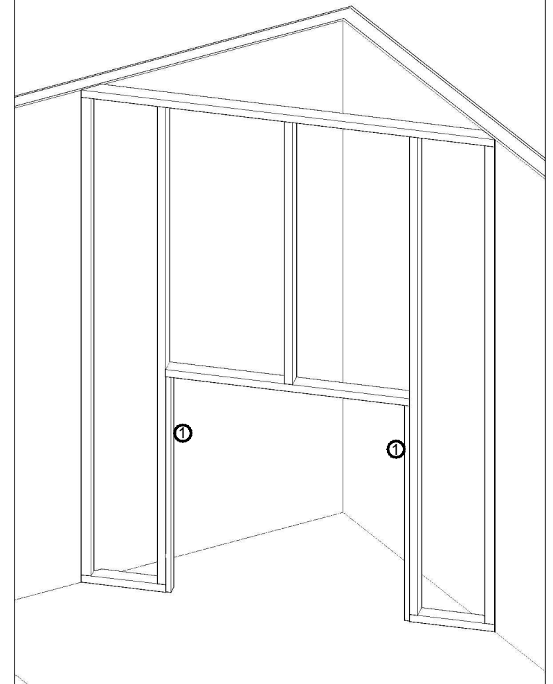
① 23 x 48 mm lekt som er festet 6 mm innenfor ytterkant av reisverk.
