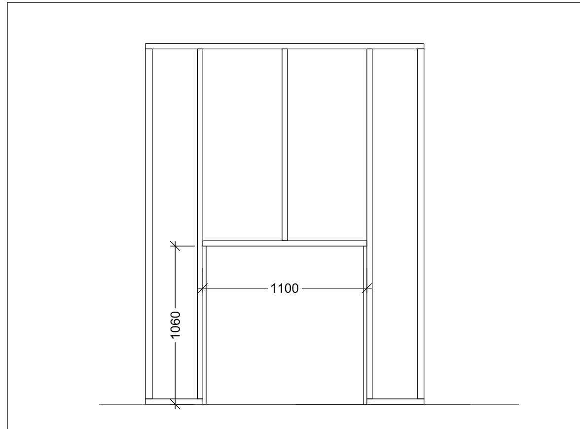
① 23 x 48 mm lekt som er festet 6 mm innenfor ytterkant av reisverk.
